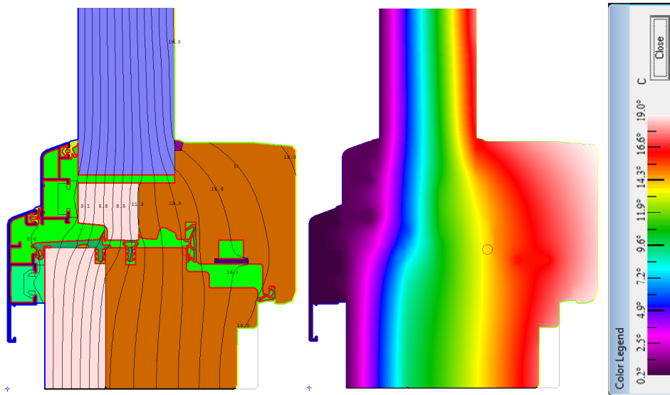
Obr. 2 Zobrazenie priebehu izoterm a infračervený priebeh teplôt v spodnom profile okenej konštrukcie
