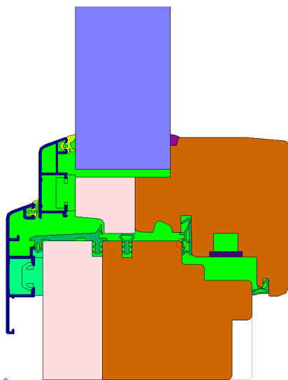
Obr. 1 Znáznornenie materiálov konštrukcie okna ALU 1083 PASSIV
